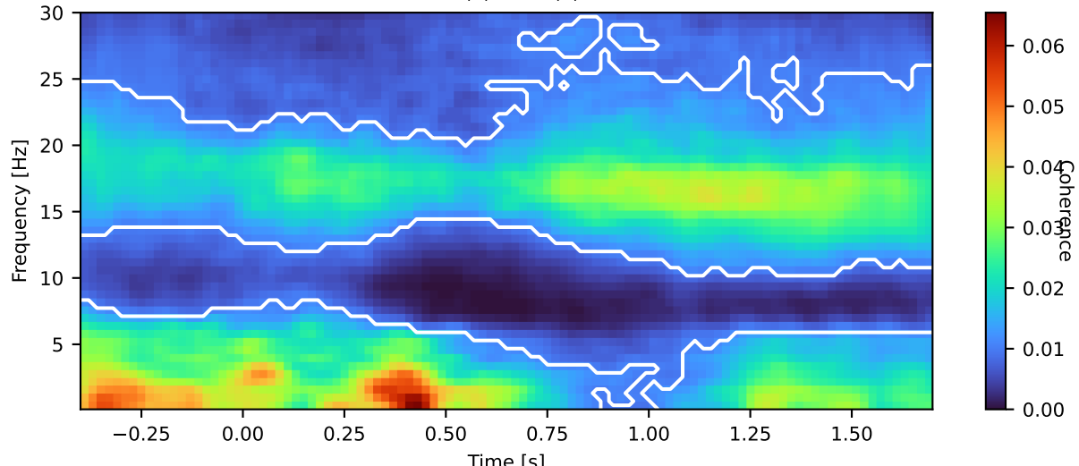
8B (0) - PEC (8)
